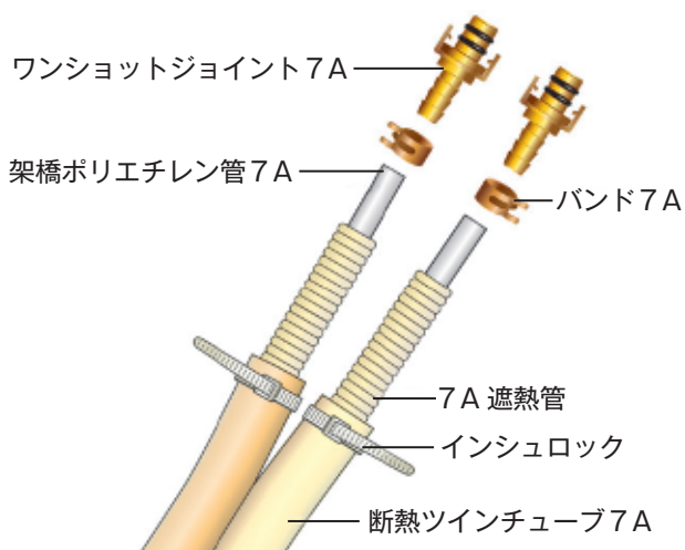
HTP-1015PT の配管図です。
